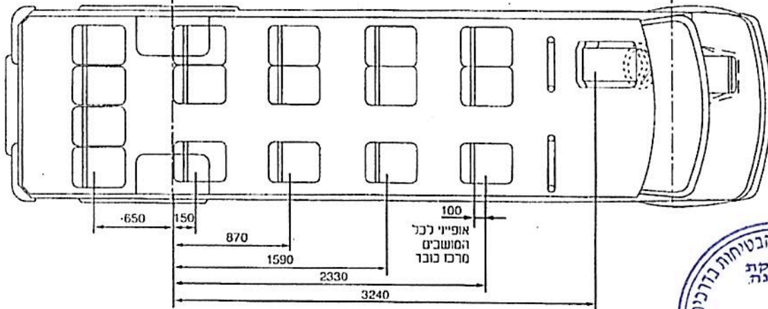
טבלת חלוקת עומסים על הסרנים
